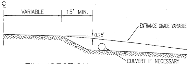
FILL SECTION
